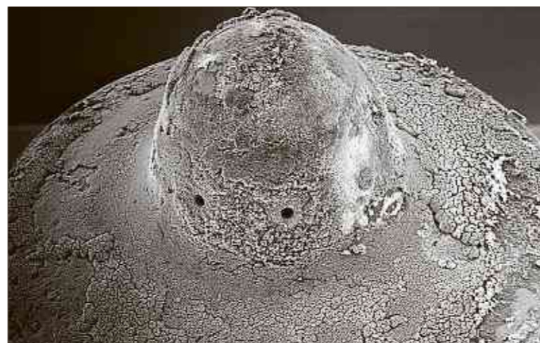
Oben eine verschmutzte Diesel-Einspritzdüse, unten ein gereinigtes Exemplar (65-fach vergrößert unter dem Rasterelektronenmikroskop).
